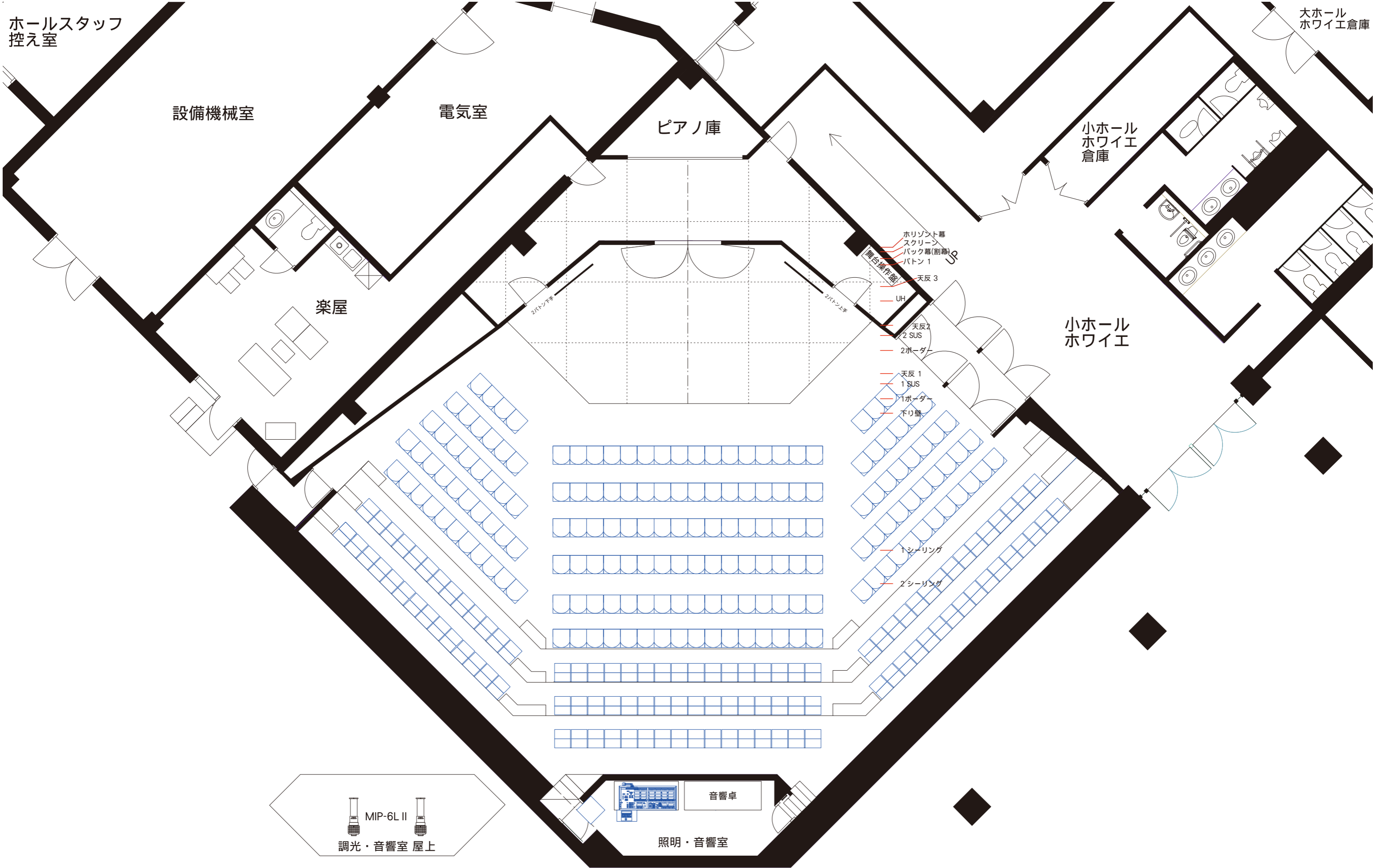
真岡市民会館 小ホール 平面図
